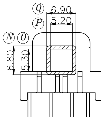
SEC. A-A
