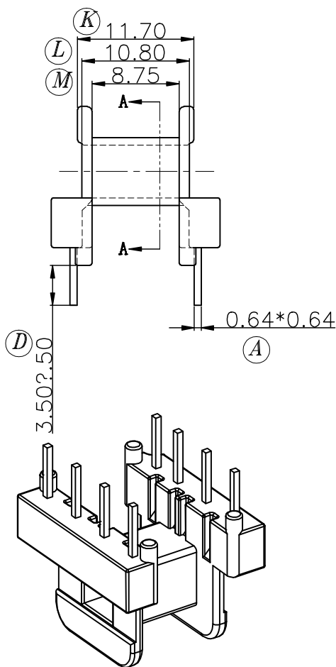
SEC. A-A
