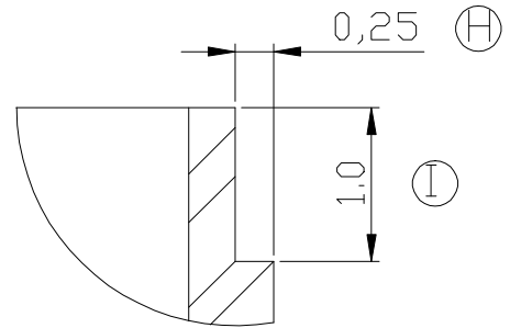
详细视图B 4:1
